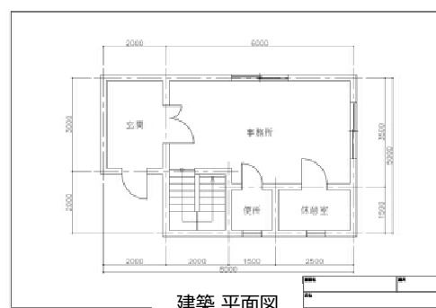
建築 平面図
